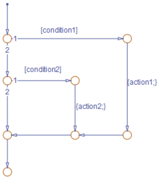
if-elseif
